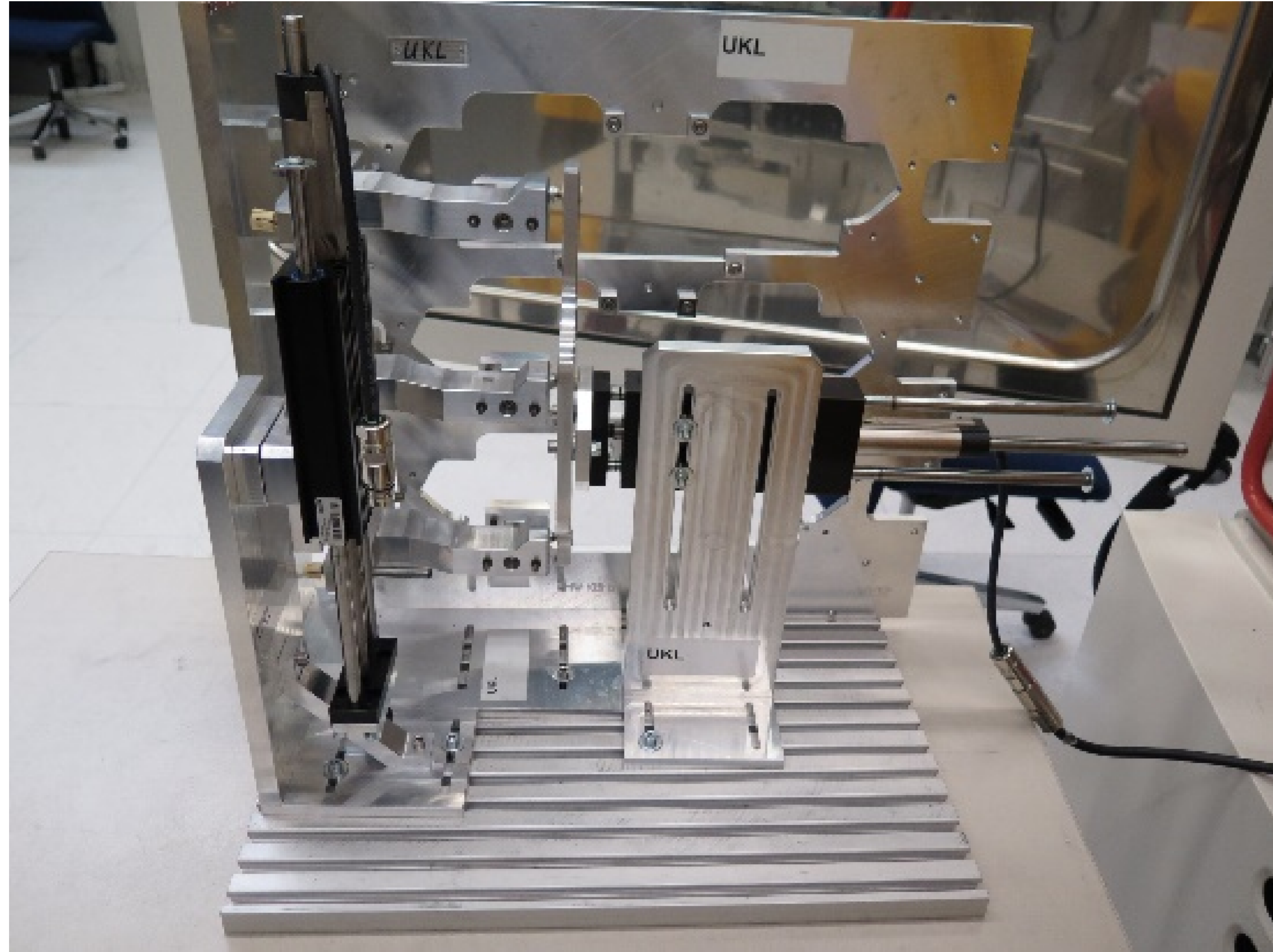
Abb.1: 3-fach Dauerlauf
